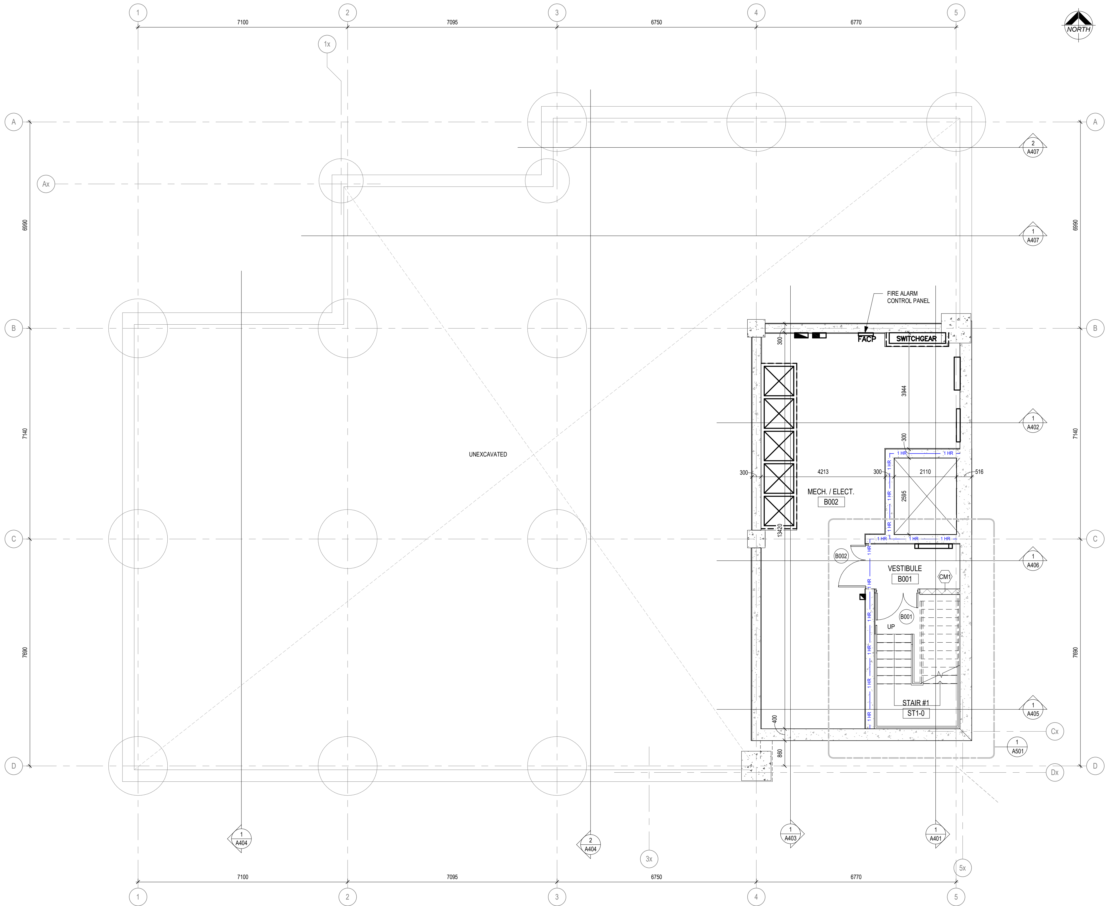
1 A201 BASEMENT PLAN 1 : 75
