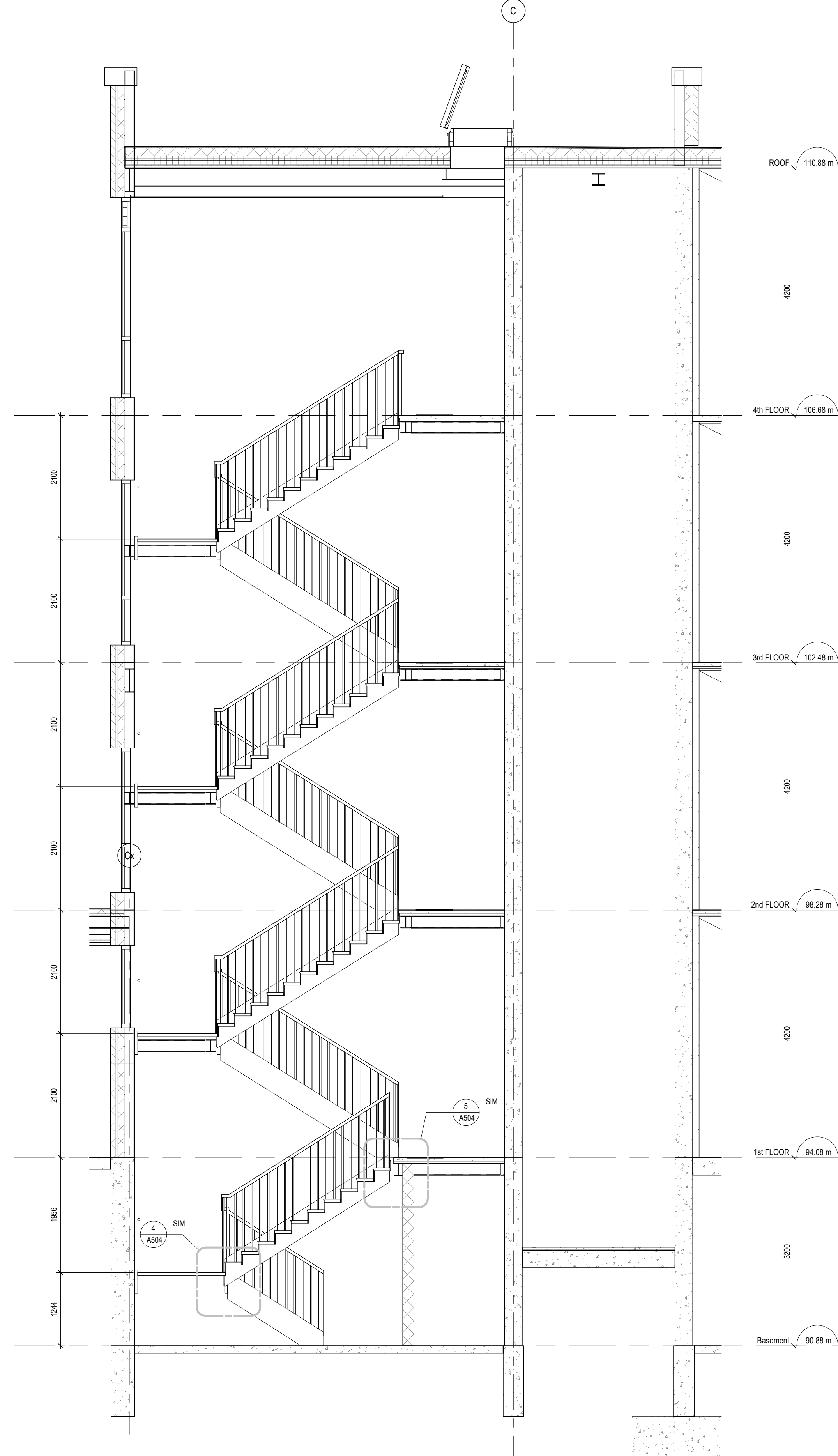
1 A502 STAIR SECTION 1 : 50
