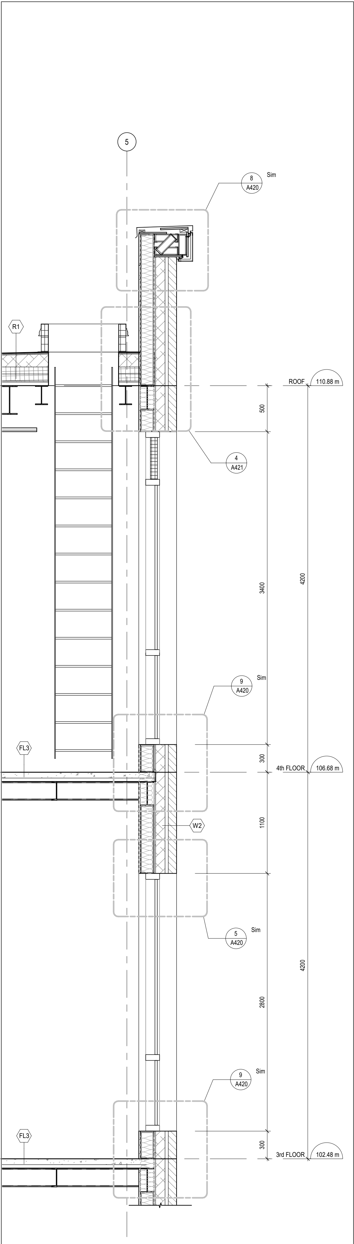
2 WALL SECTION 1 : 25
