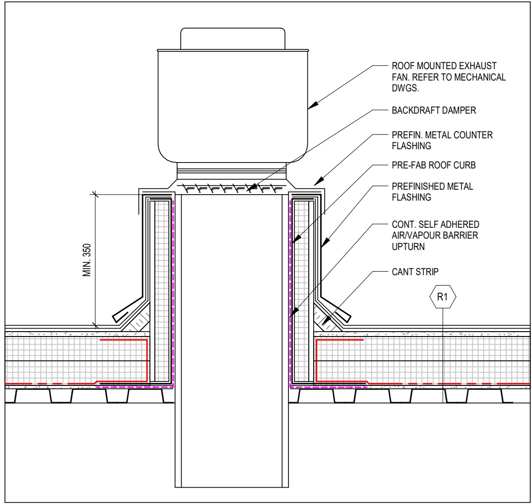
5 TYP. VENT EXHAUST FAN DETAIL A206 1 : 10
