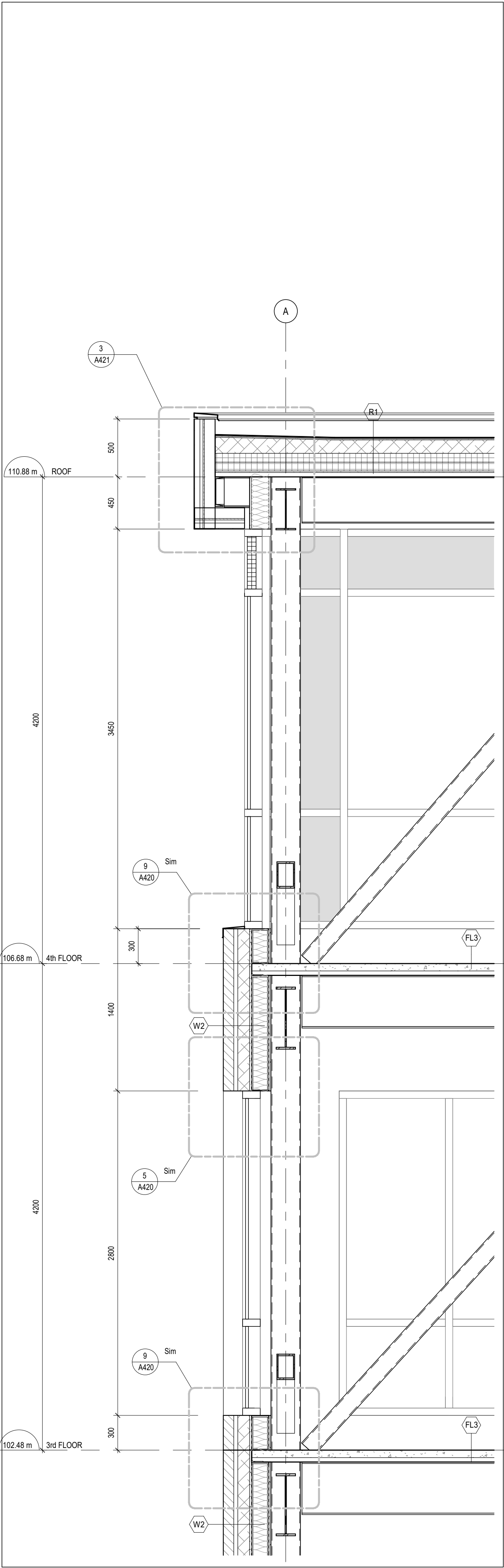
1 WALL SECTION A411 1 : 25
