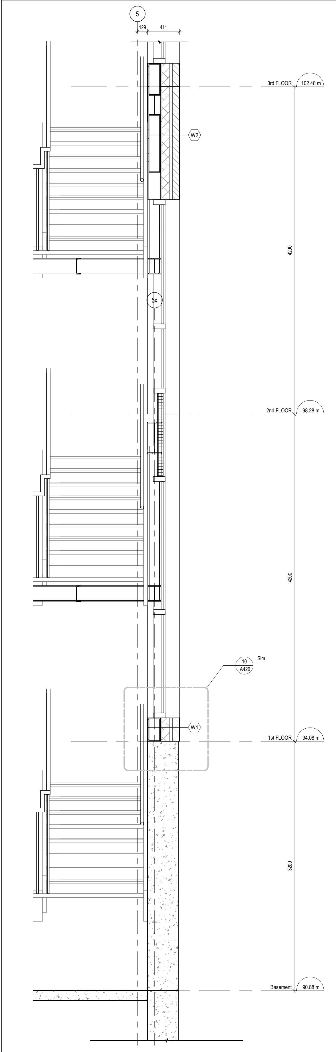
3 WALL SECTION A413 1 : 25
