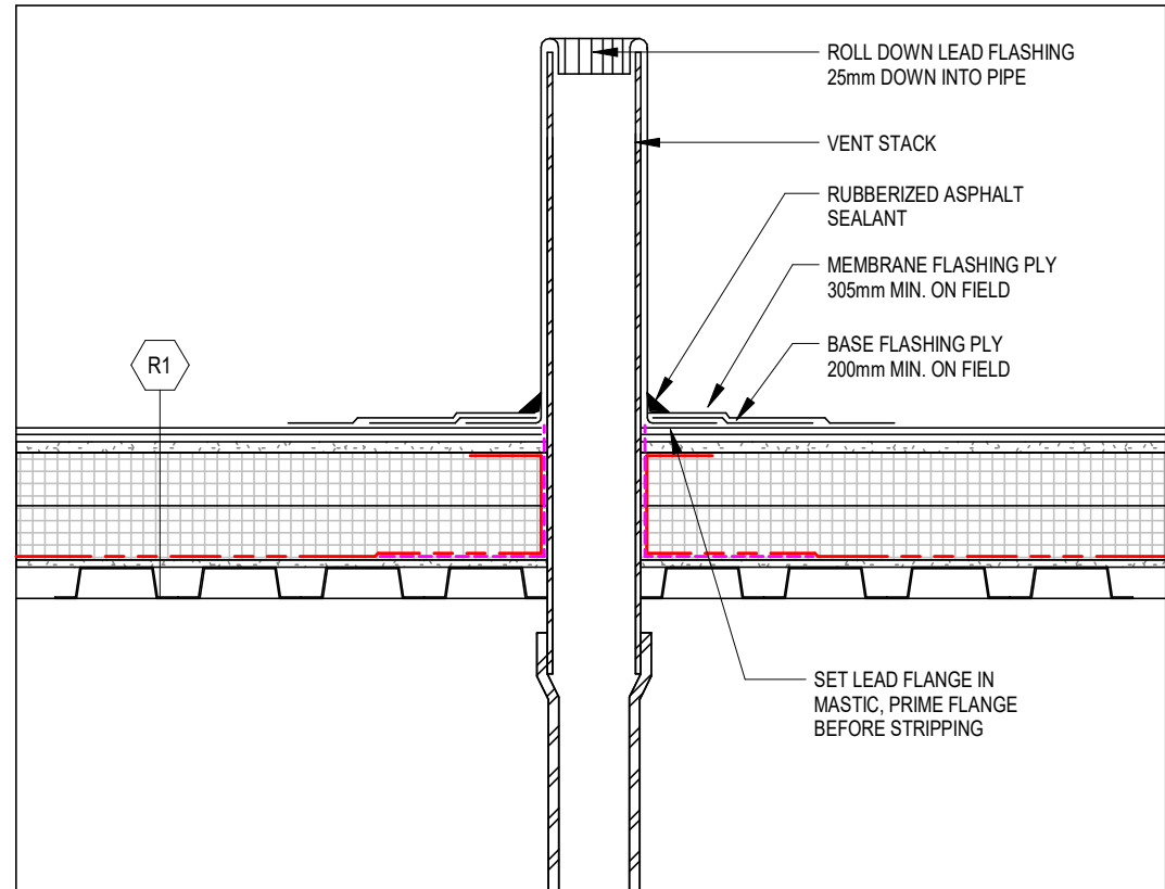
2 TYP. VENT STACK DETAIL A206 1 : 10
