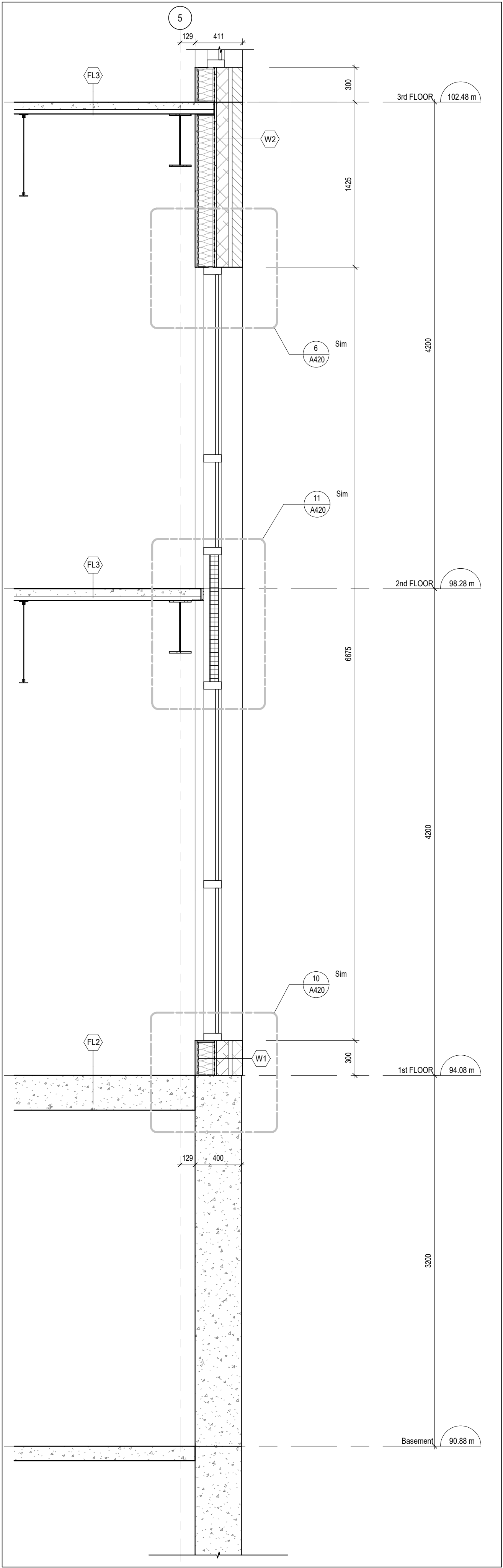
2 WALL SECTION A411 1 : 25
