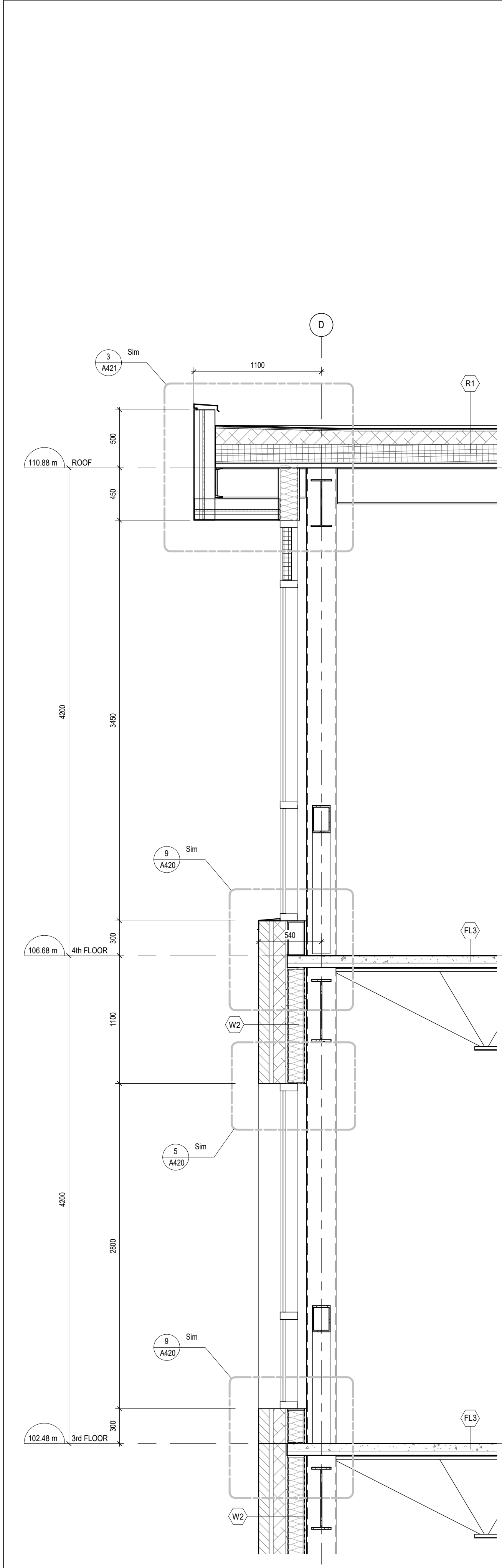
2 WALL SECTION A413 1 : 25
