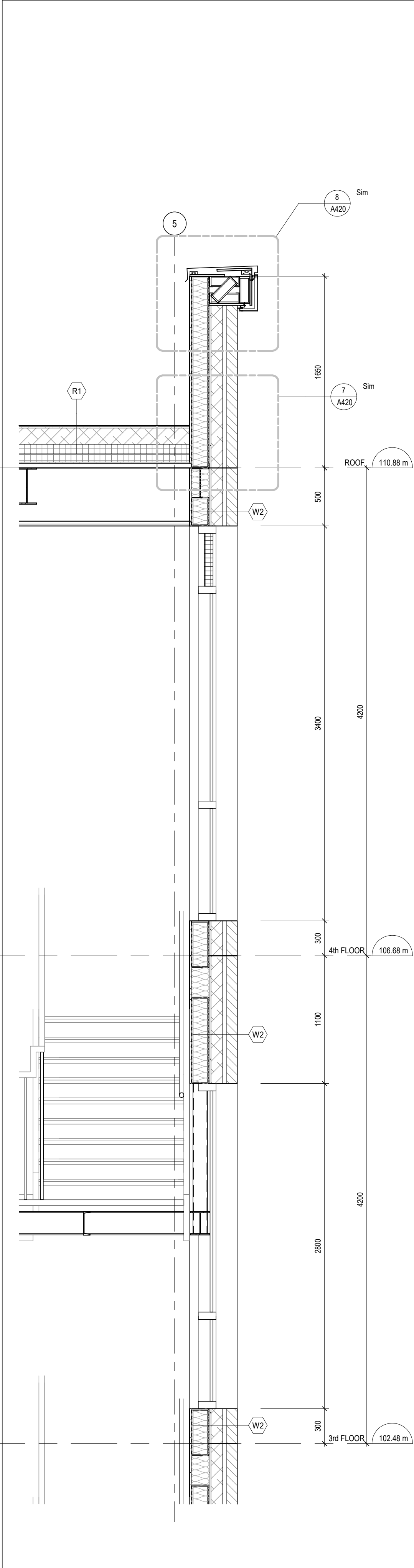
4 WALL SECTION A413 1 : 25
