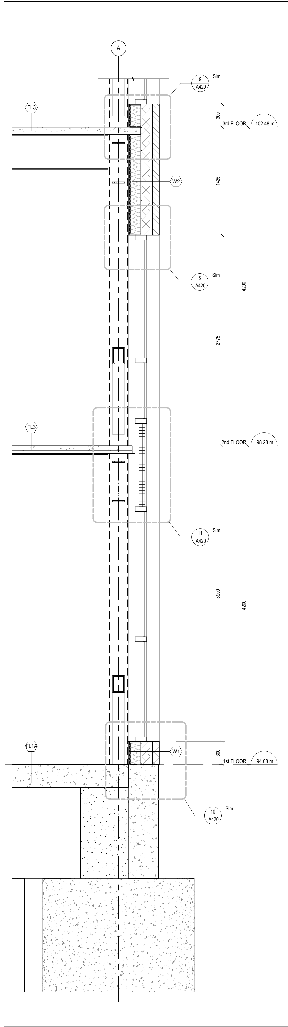
4 WALL SECTION A411 1 : 25
