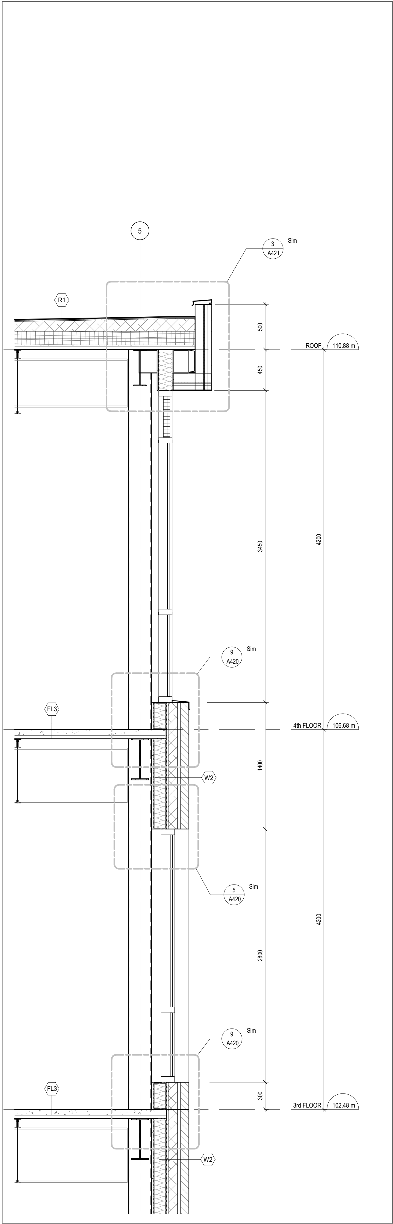
3 WALL SECTION A411 1 : 25
