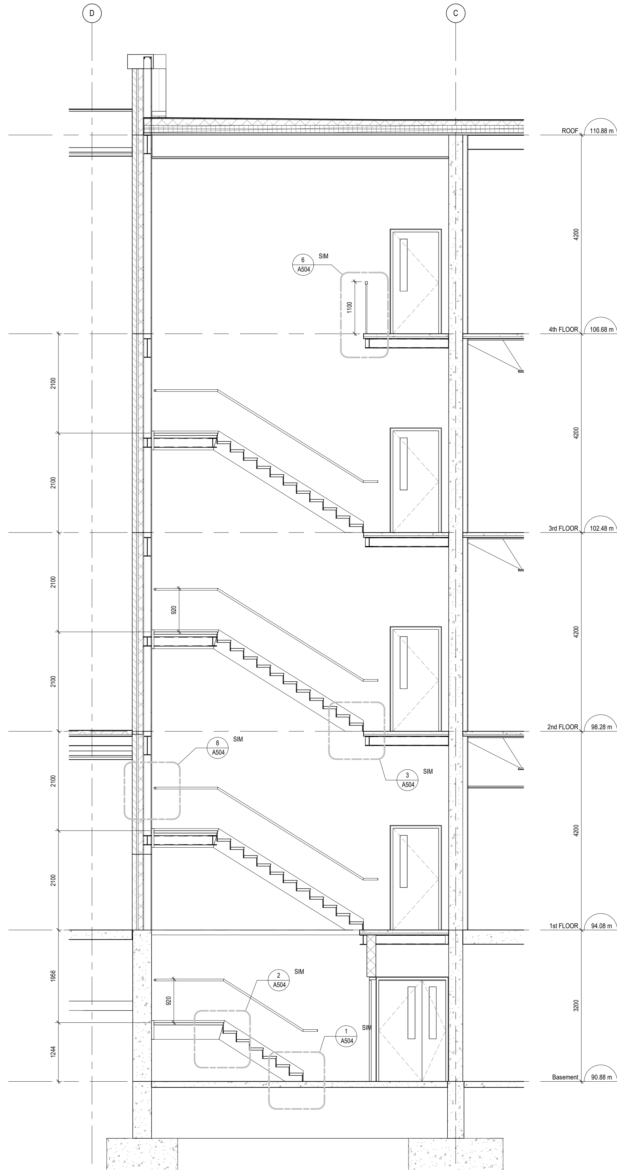
2 A502 STAIR SECTION 1 : 50
